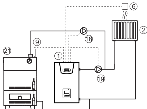
Рис.7 Упрощенная схема подключения котла в режиме вспомогательного.
